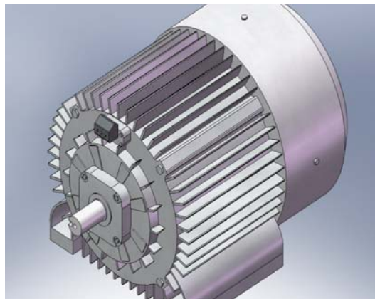
FIG. 1, CARCAZA EXTERNA DEL MOTOR, VISTA ISOMÉTRICA.
